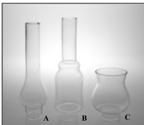
A) 143/24 (Ø3,5xØ7xØ4x h.24) B) 144/26 (Ø3,5xØ8xØ5x h.26) C) 142/12 (Ø8xØ10xØ5x h.12) Corte Frío
