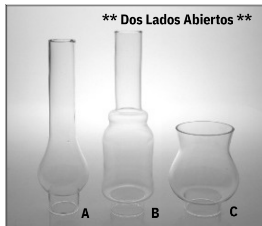
A) 143/27 (Ø3,5xØ9xØ6x h.27) B) 144/26 (Ø3,5xØ8xØ5x h.26) C) 142/12 (Ø8xØ10xØ5x h.12) Corte Frío
